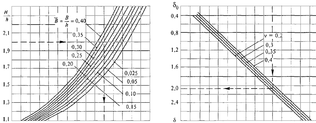
Рисунок Ж.1 - Номограмма для определения значений \delta_0
