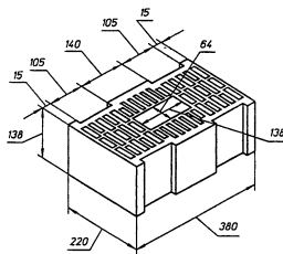
Рисунок А26 — Камень с пустотностью 55 %
