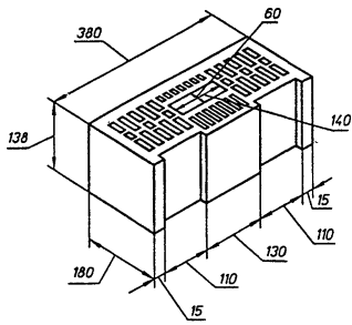
Рисунок А23 — Камень с пустотностью 45 %
