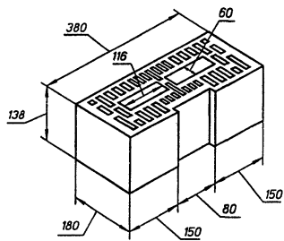
Рисунок А24 — Камень с пустотностью 55 %
