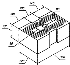
Рисунок А25 — Камень с пустотностью 45 %
