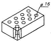
Рисунок А13 — Кирпич с 11 сквозными отверстиями (пустотность 8,2 %)
