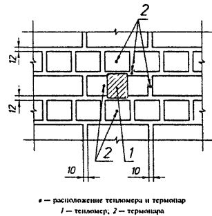
Рисунок 1 – Техническая характеристика фрагмента кладки
