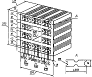
Рисунок А19 — Камень с 10 отверстиями и одной или двумя продольными канавками
