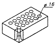
Рисунок А14 — Кирпич с 17 сквозными отверстиями (пустотность 12,7 %)
