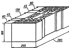
Рисунок А27 — Камень с пустотностью 55 %
